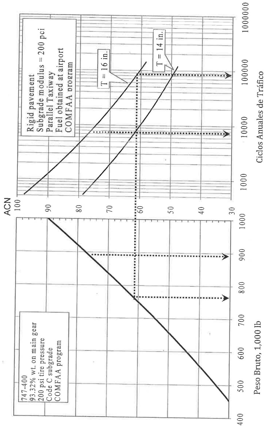
Figura A3-6. Vida Útil de Pavimento para B747-400
